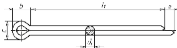
DIN94
