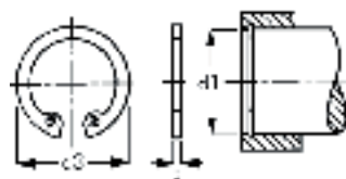
DIN 472
