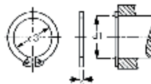
DIN 471
